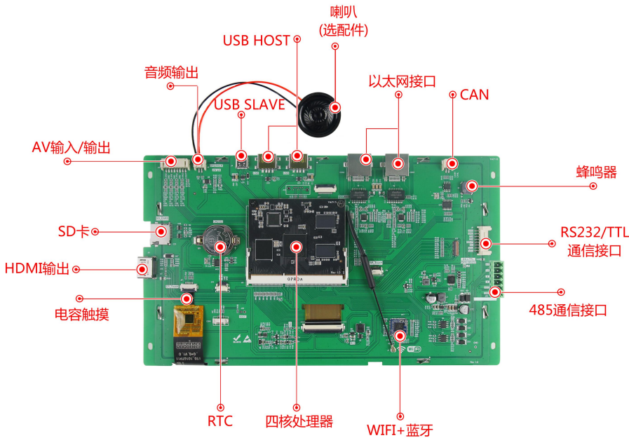
图 1-2 硬件配置图
